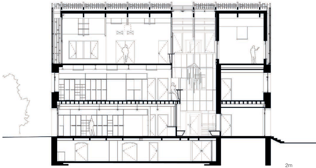
Coupe longitudinale
