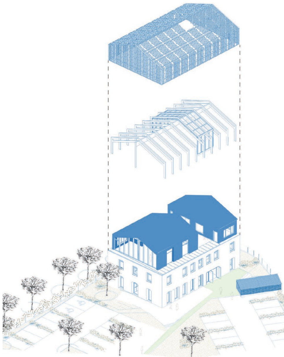
Axonométrie éclatée de la restructuration
